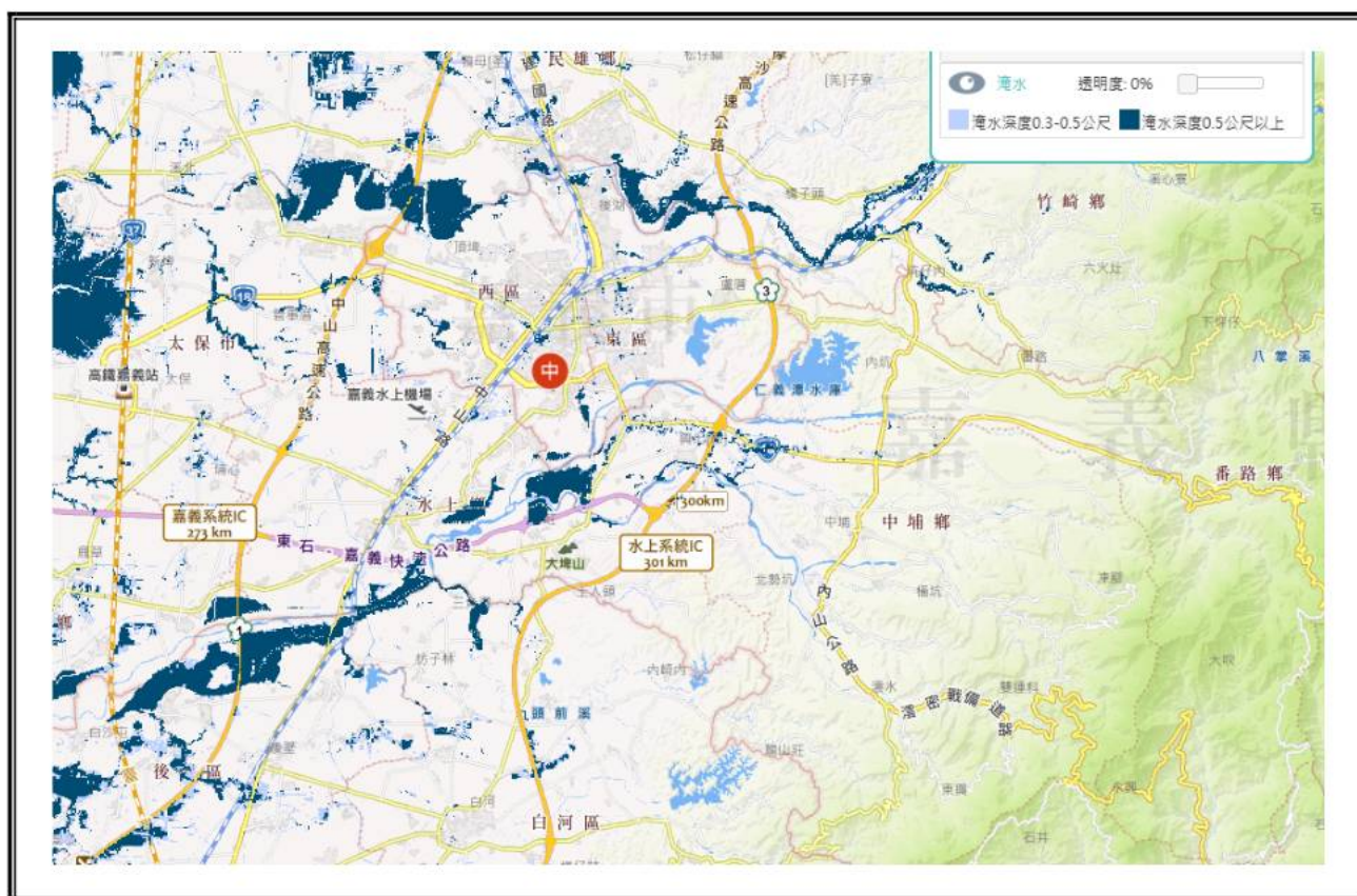
圖 2.4.2 淹水災害潛勢圖 (瀏覽日期： 113 年 10 月 8 日)
