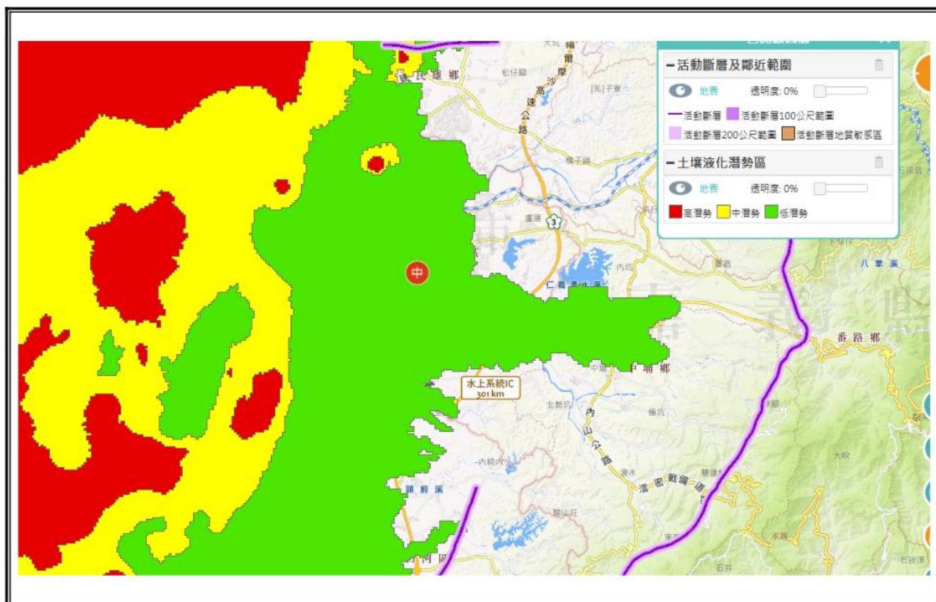
圖 2.4.1 地震災害潛勢圖 (瀏覽日期： 113 年 10 月 8 日)
