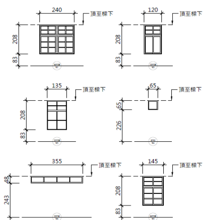
① 一層平面圖 (廚房) SCALE A1:1=50; A3:1=100
