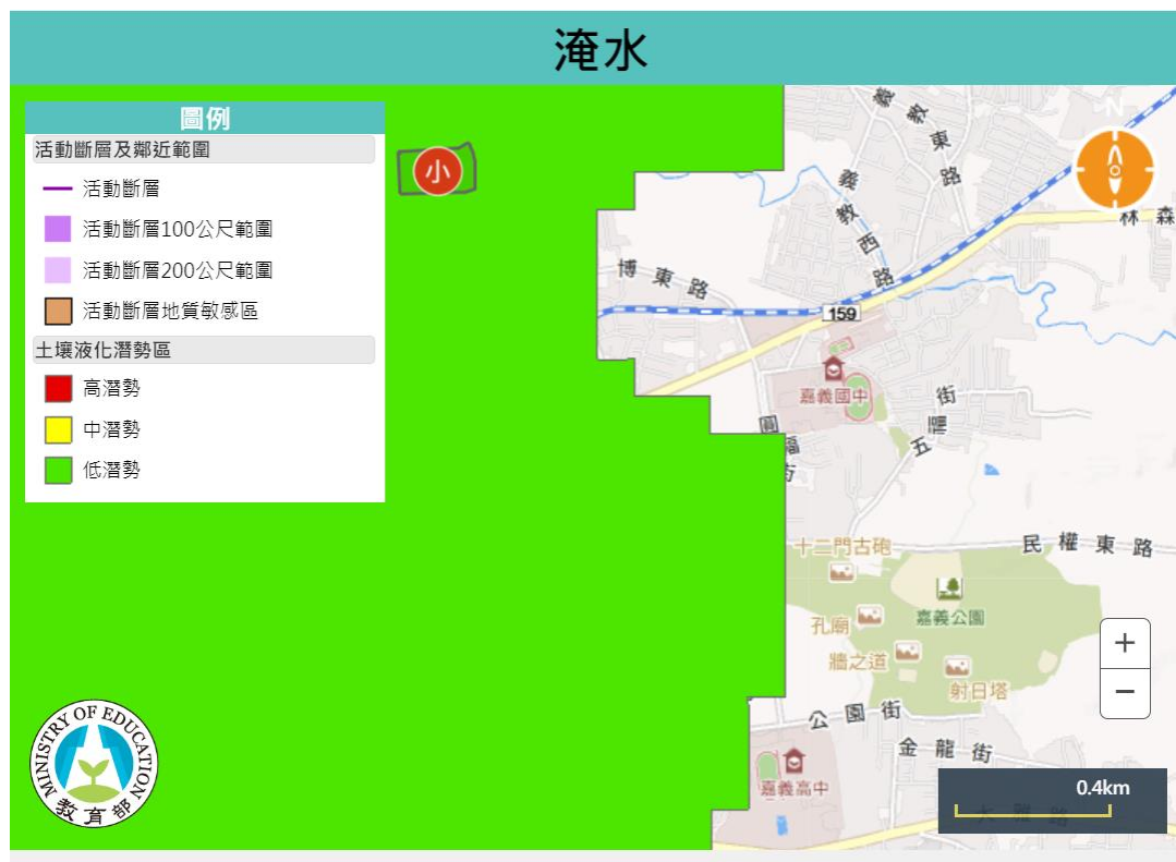
圖 2.4.1 地震災害潛勢圖 (瀏覽日期：113 年 8 月 21 日)
